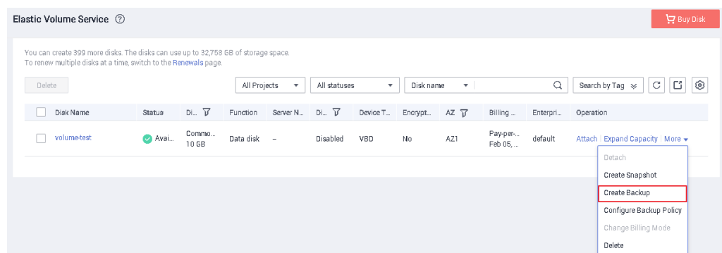
Figura 9-2 Criar backup
