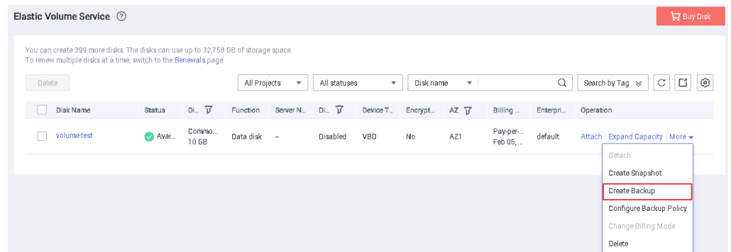
Figura 5-2 Criar backup
