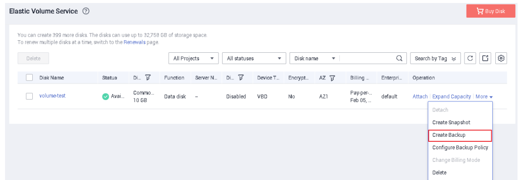
Figura 2-1 Criar backup
